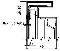
Section:A-A'(S:3/1)
